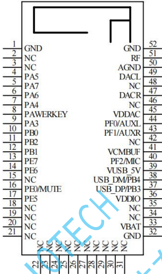
ANS-BT301S 引脚定义图（顶视图）
