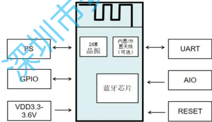
ANS-BT301S 框图（顶视图）
