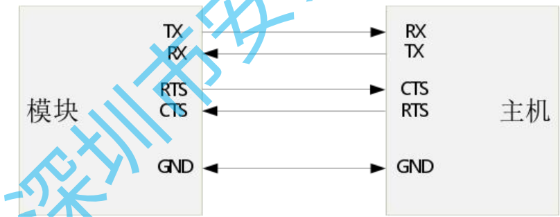
模块与主机连接图
