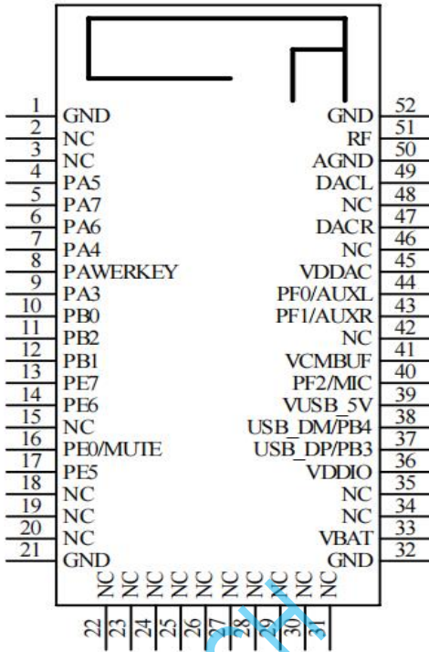
ANS-BT301S 引脚定义图（顶视图）
