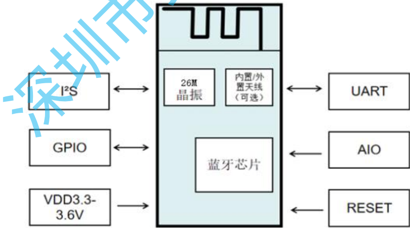
ANS-BT301S 框图（顶视图）
