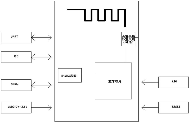
ANS-BT102S 框图（顶视图）
