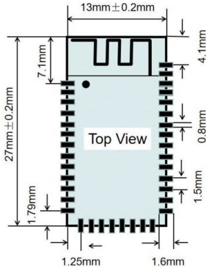
ANS-BT102S 封装（顶视图）
