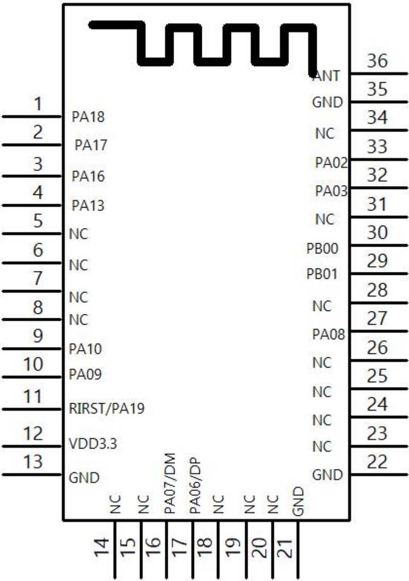
ANS-BT102S 引脚定义图（顶视图）
