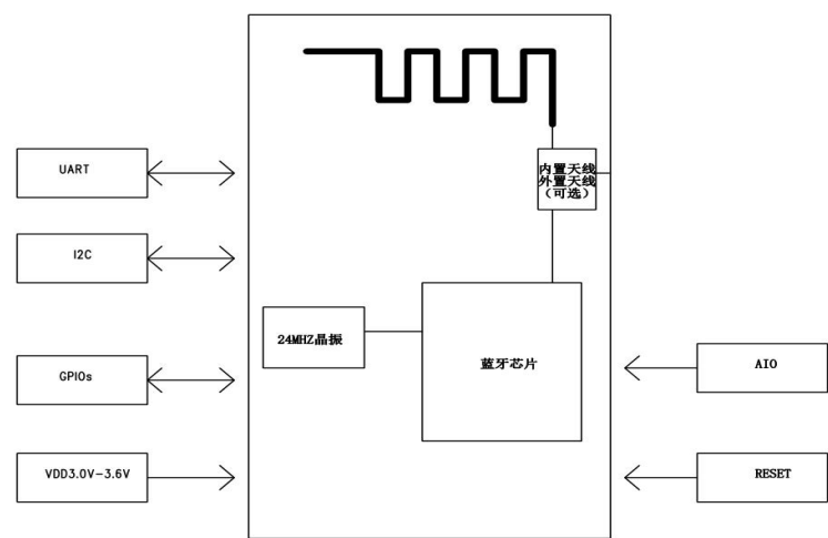
ANS-BT102M 框图（顶视图）
